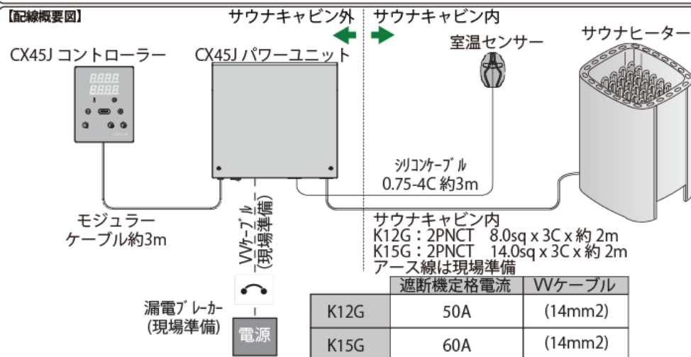
【配線概要図】
