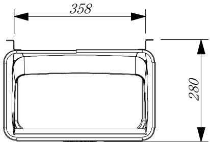
上面図
