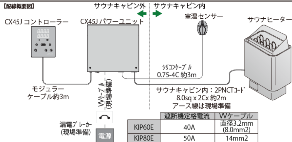
【配線概要図】
