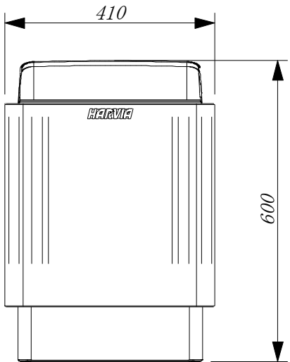
正面図
