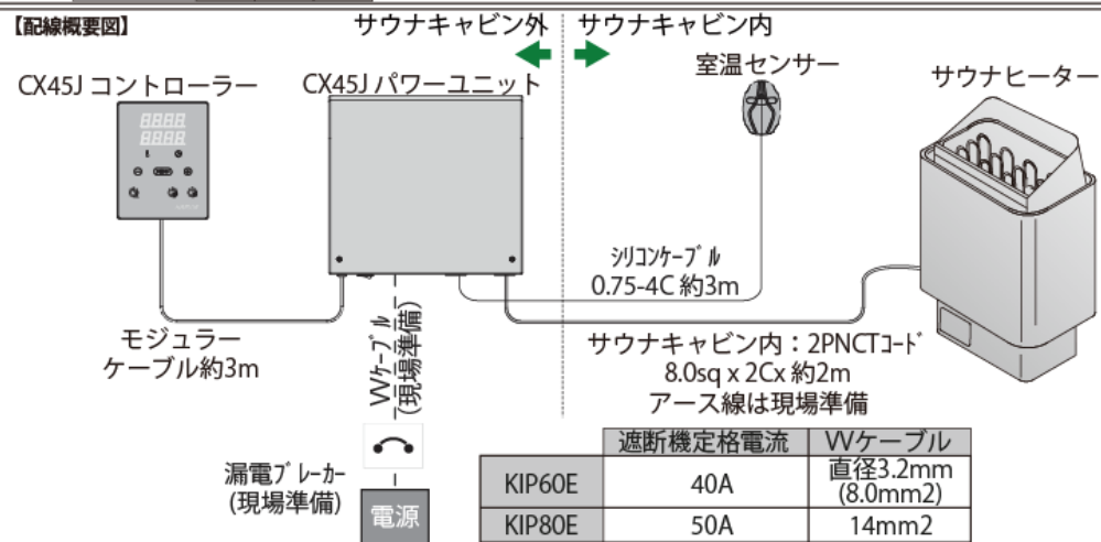
【配線概要図】
