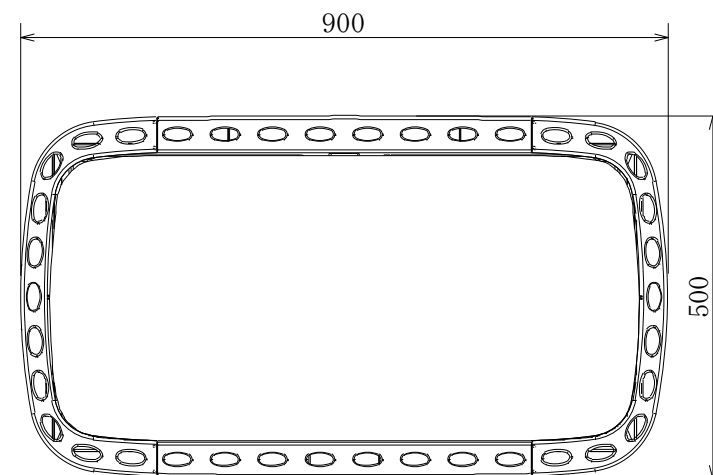
上面図
