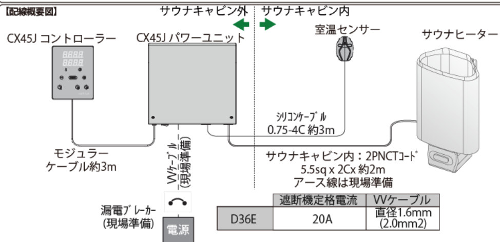
【配線概要図】
