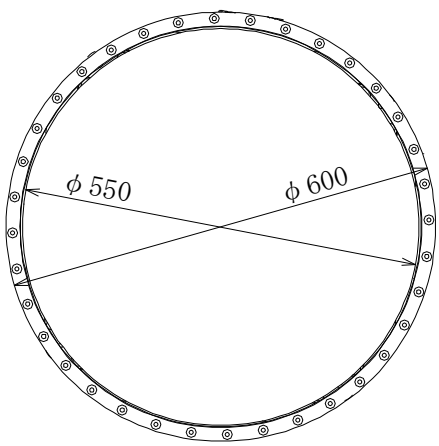
上面図
