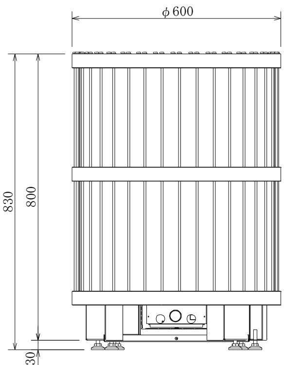
正面図
