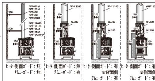
Case2: タイルフロアーの場合
