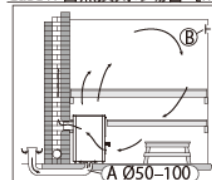
Case1: 自然換気の場合 [mm]
