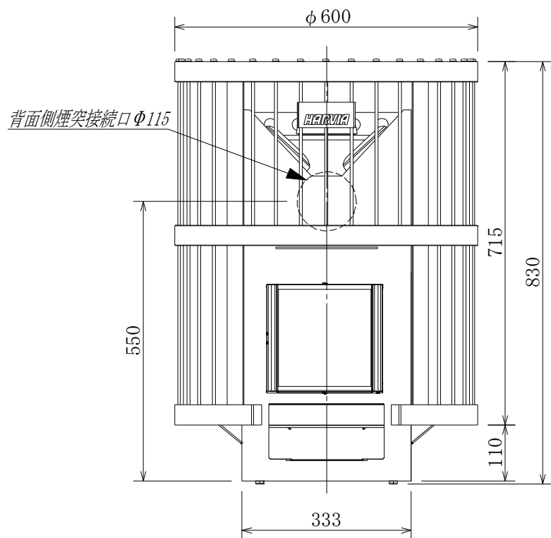
正面図
