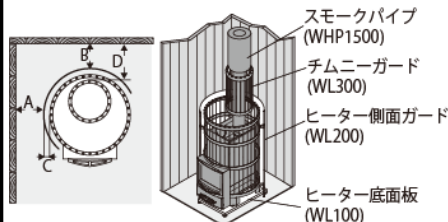
Case2: ヒーター側面ガード (WL200) とチムニーガード (WL300) を使用する場合の最低離隔距離 [mm]
