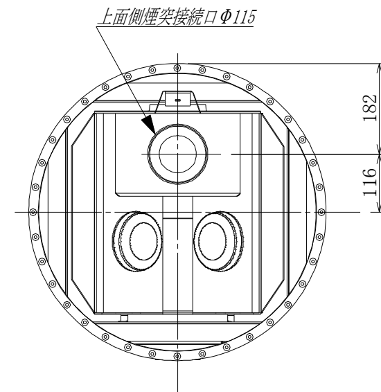
上面図
