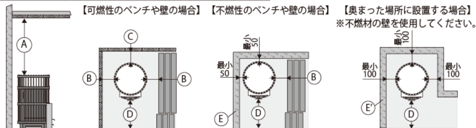
Case1: ヒーター側面ガードを使用しない場合の最低離隔距離 [mm]
