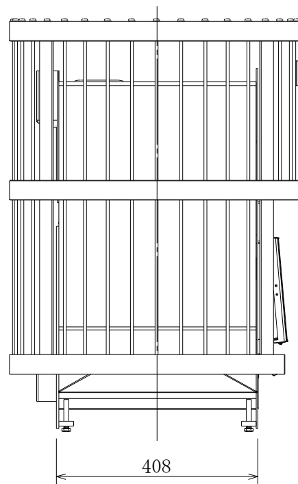
側面図
